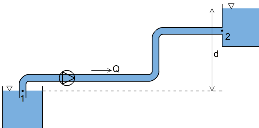
Σχήμα 1: Ένας καταθλιπτικός αγωγός μεταφέρει παροχή Q από μία δεξαμενή χαμηλού υψομέτρου σε μία υψηλή. Το γεωμετρικό ύψος του συστήματος είναι d .
